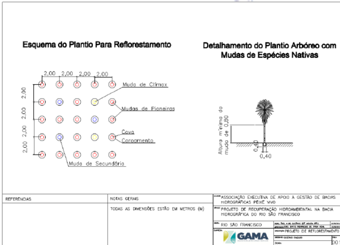
Figura 20: Especificações técnicas para execução do plantio das mudas na área da sub-bacia do Córrego do Marinheiro
